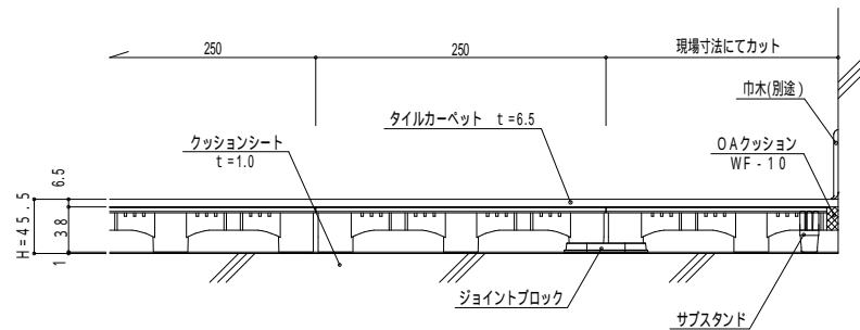
断面図 S = 1 : 5
